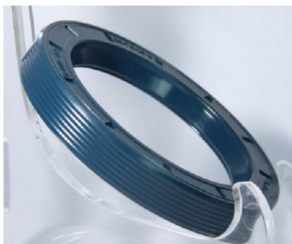
Abbildung 1: Neue verbesserte Radialwellendichtung 12010969B mit Rillen für eine bessere Dichtwirkung
